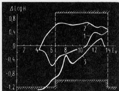
РИС. 2. График суммарной погрешности экспозиции ( \Delta \log H ): 1 — «Пентакс-МХ» № 4246294; 2 — «Зенит-автомат» № 8604516; 3 — «Зенит-автомат» № 8600523. \delta p_1=1,05 ст; \delta p_2=0,9 ст; \delta p_3=1,5 ст.
